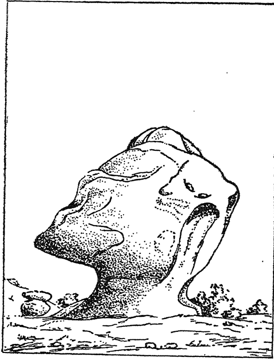
चित्र २००—मशरूम ग्रेनाइट, जोधपुर, राजस्थान मरुस्थल
